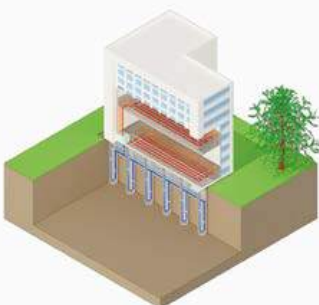
Pompe à chaleur sur géostructures énergétiques
